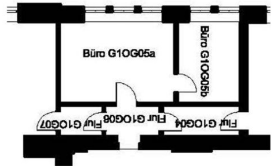
Zweiraumbüro-Galerieebene-Lohnhalle-G10G05_Grundriss
